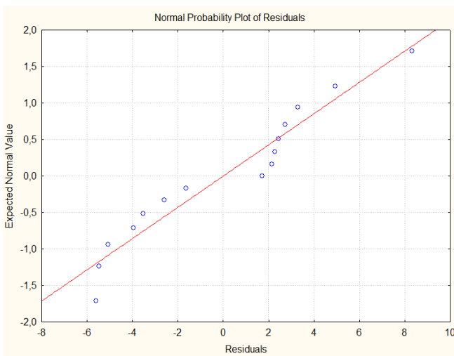
Рис. 1.5. а) Окно предсказаний в программе Statistica; б) Результат построенной модели; в) Нормальный вероятностный график остатков
