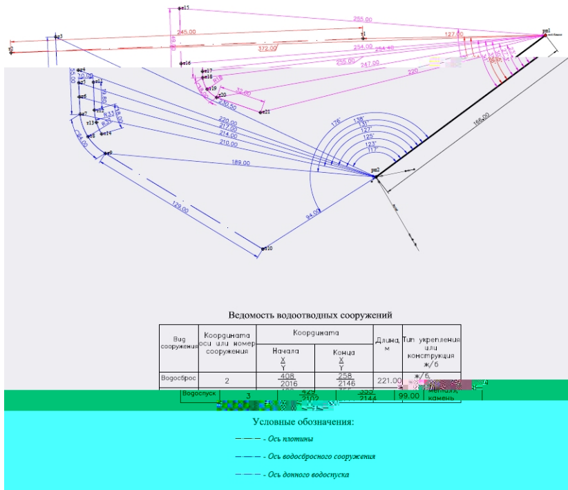
Рис. Разбивочный план
