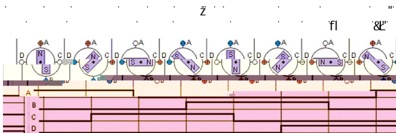
Рис. 2. Управление в полушаговом режиме
