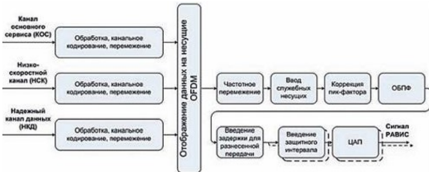
Рис. 1. Структурная схема передающей части РАВИС
