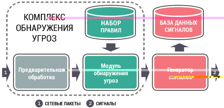
Рис. 1. Общая схема IDS (системы обнаружения вторжений)
