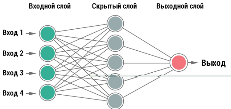
Рис. 2. Структура ИНС (с одним скрытым слоем)
